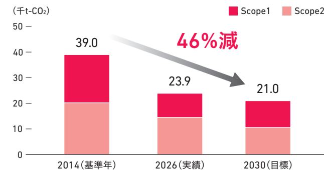
●CO 2 排出量(各年3月期)
